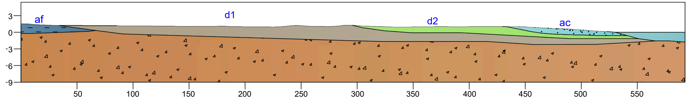
SEZIONE GEOLOGICA A - B
