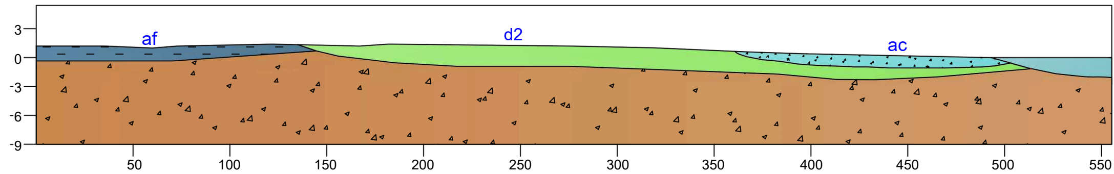
SEZIONE GEOLOGICA C - D
